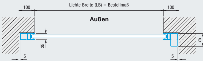
Einbau hinter der Öffnung
