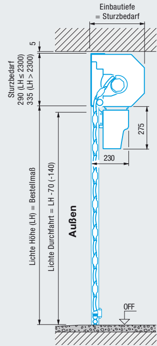
Einbau in der Öffnung
