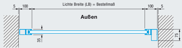
Einbau in der Öffnung
