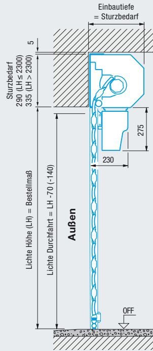
Einbau hinter der Öffnung
